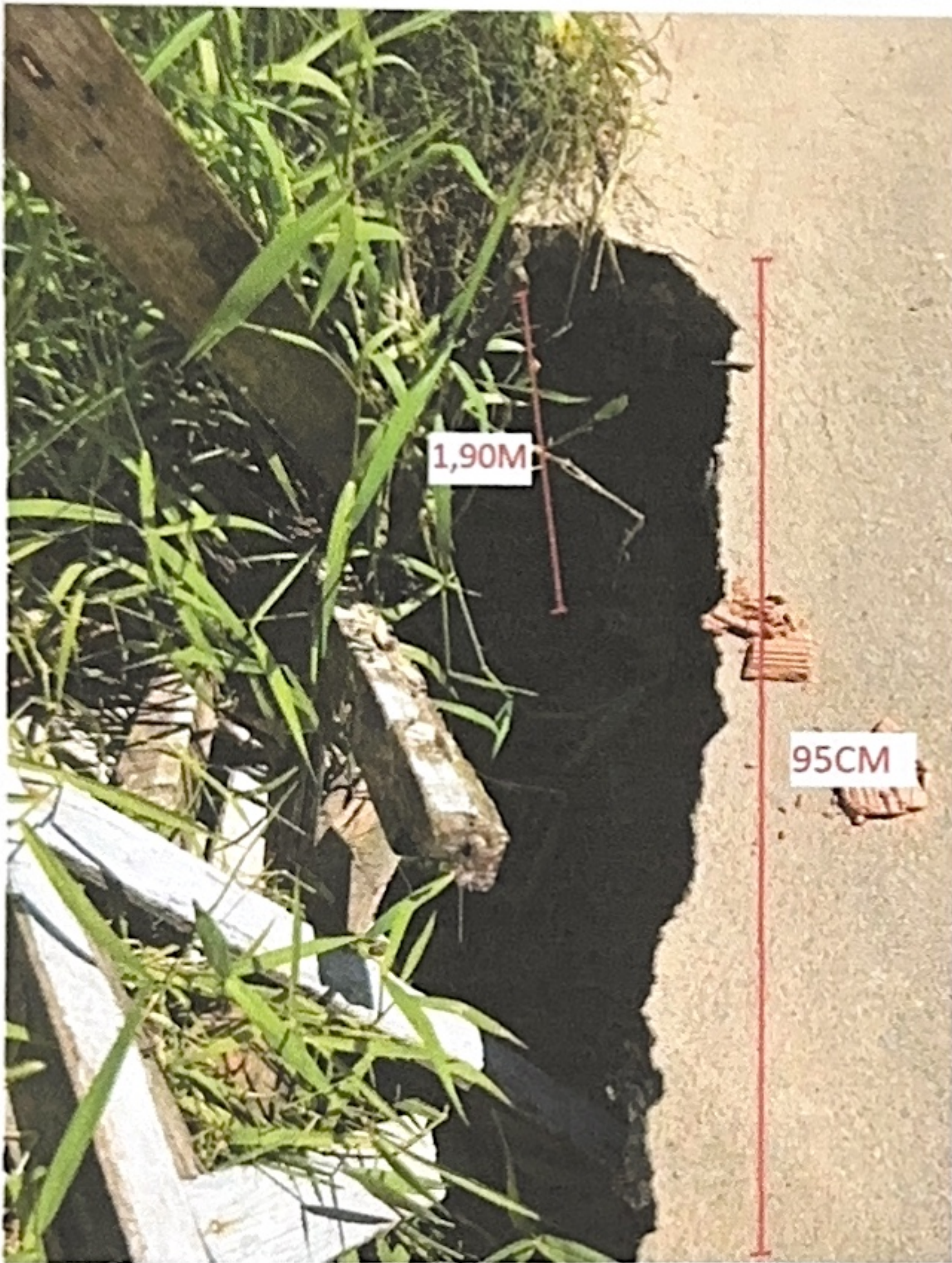
Figura 5: Buraco-2 especificado com suas dimensões.
